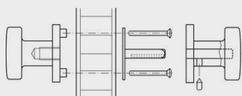
Verschraubung: Gegenseitig GGV Art.-Nr.: 3212 GGV & 3214 GGV
