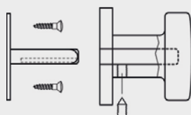
Verschraubung: Einseitig ENV Art.-Nr.: 3213 ENV & 3215 ENV
